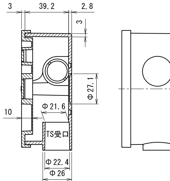
断面 A-A
