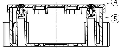
断面 B-B
